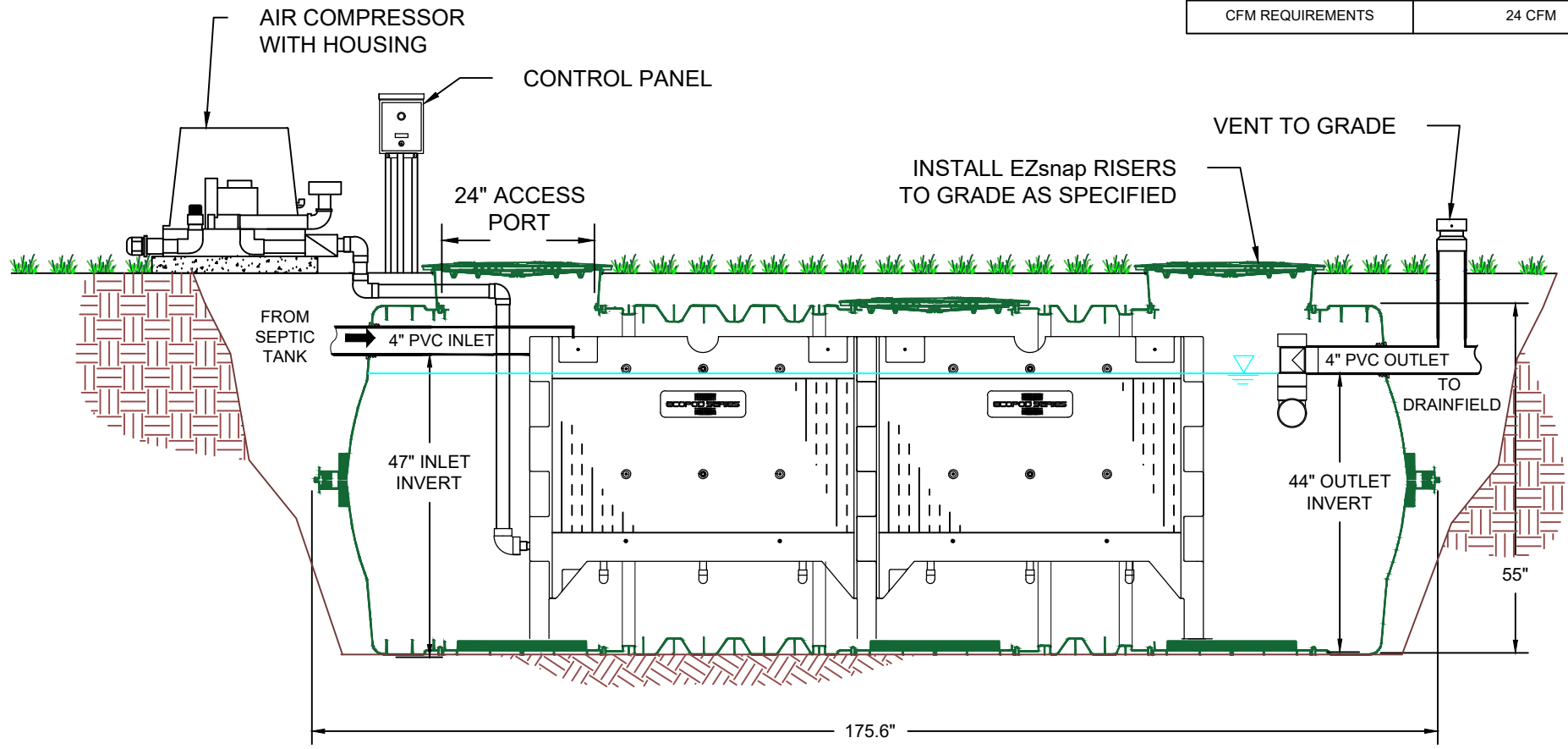
E100-N IM-1530 REACTOR TANK
