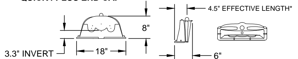
QUICK4 PLUS END CAP
