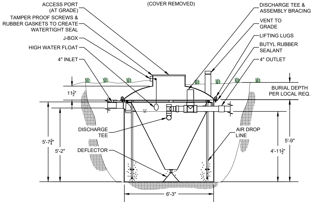
SECTION A-A
